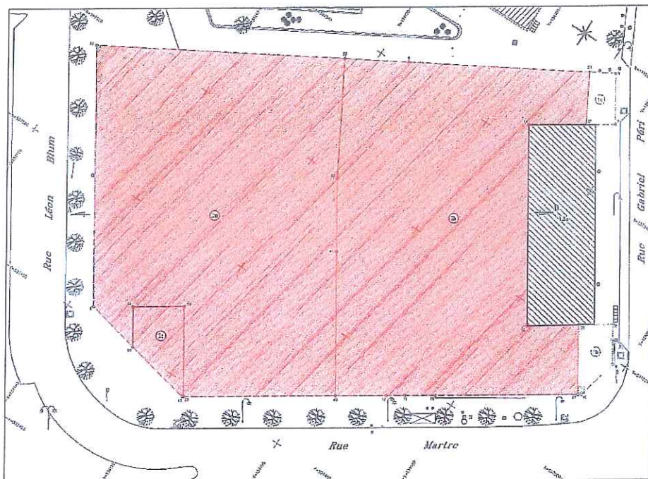
Figure 3 : Sous-sol du centre Léon Blum (volume 1 000 en jaune ; volume 2 000 en rouge)
