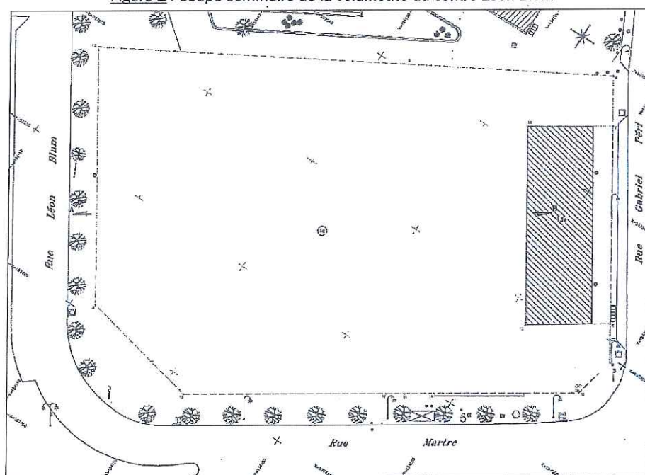
Figure 2: Tréfonds du centre Léon Blum (volume 1 000 en jaune)
