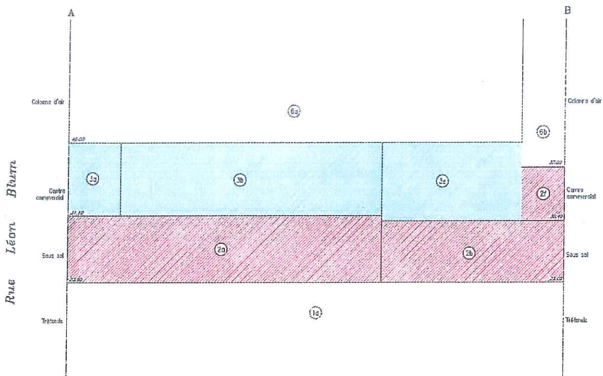
Figure 1 : Coupe sommaire de la volumétrie du centre Léon Blum (volume 2 000 en rouge)
